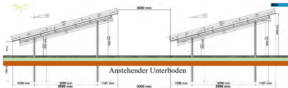
Abb.5: Technische Abmessung der aufgeständerten Solaranlage.
