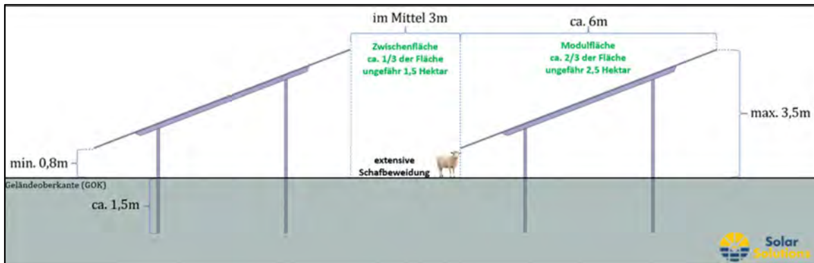
Skizze: Aufgeständertes Solarmodul ohne Fundament mit entsprechendem Bodenabstand für eine Schafbeweidung
