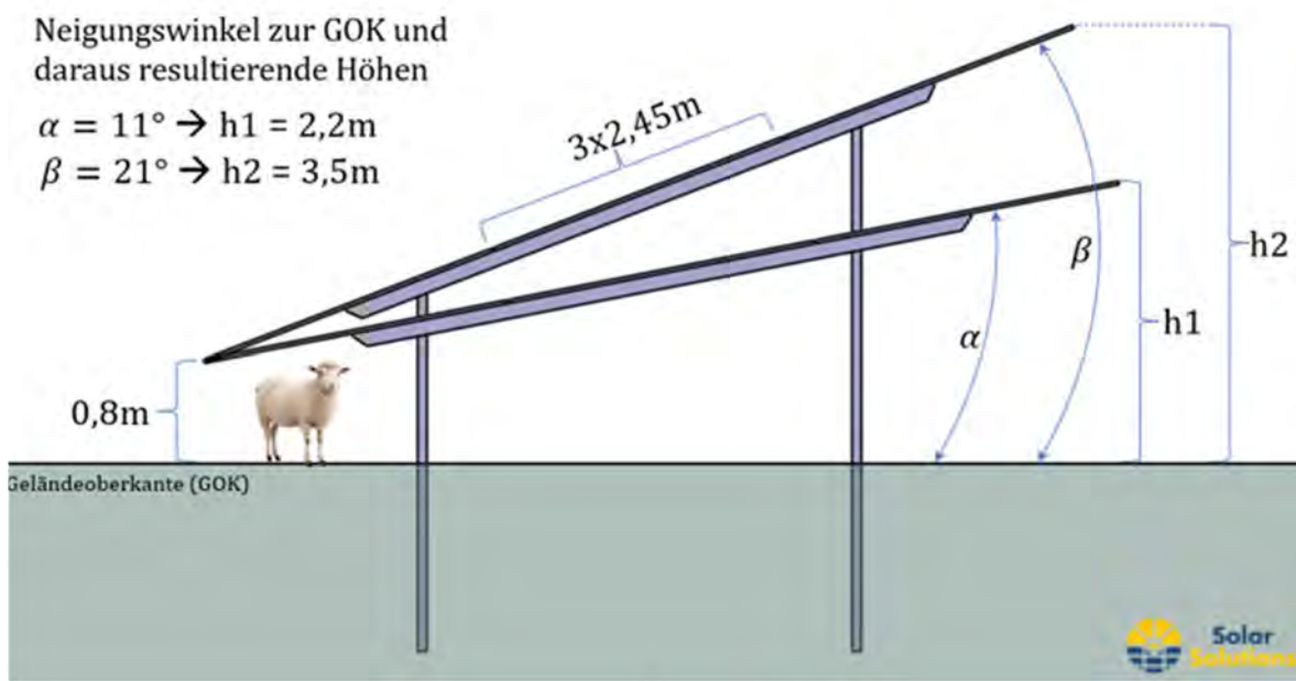
Skizze: Aufgeständertes Solarmodul ohne Fundament mit entsprechendem Bodenabstand für eine Schafbeweidung
